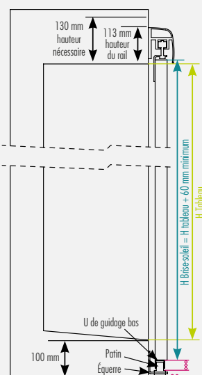
Appuis type N°7
