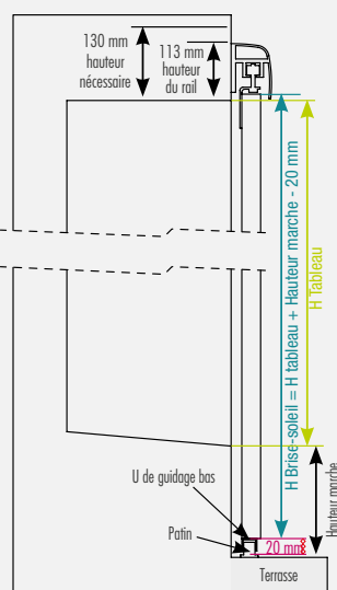
Appuis type N°8
