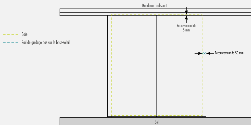
Coupe verticale du brise-soleil avec appui
