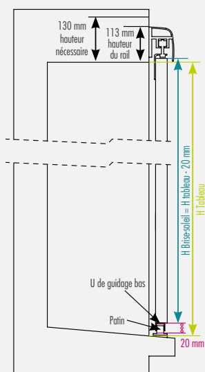
Appuis type N°5 et 6
