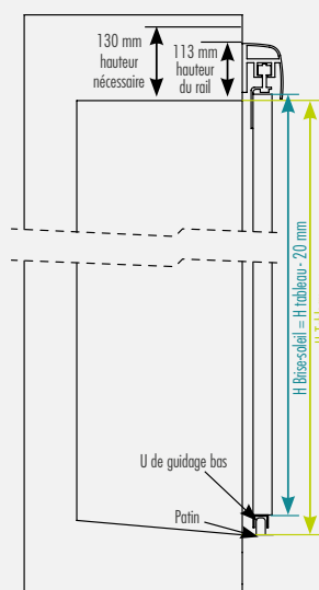
Appuis type N°9
