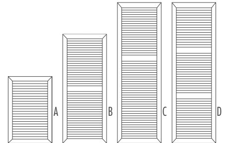
Traverse intermédiaire si hauteur remplissage > 1700 mm
