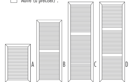
Traverse intermédiaire si hauteur remplissage > 1700 mm
