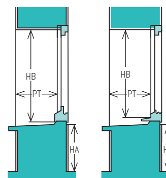
Appui traditionnel
