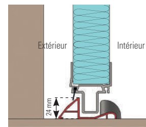
Guidage bas
