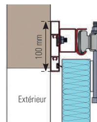
Guidage haut
